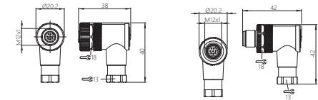
螺钉直角型母头
