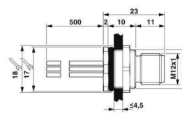
公头尺寸图
