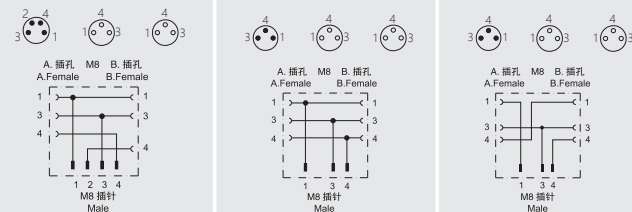
插头针脚布置及接线图
