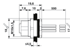
母头尺寸图
