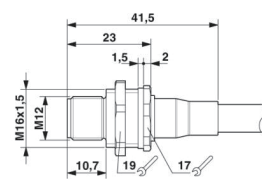
带护套 屏蔽 公头尺寸图
