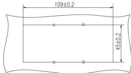
安装板开孔
