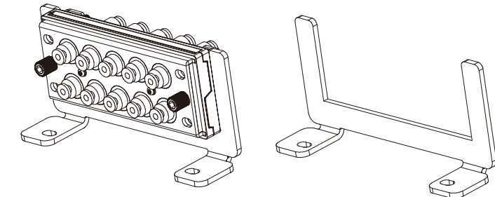
安装支架型号:8A1000
