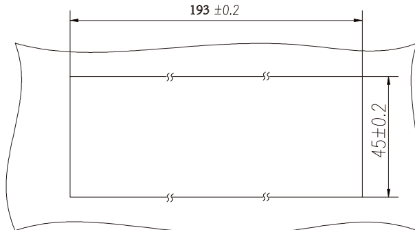
安装板开孔
