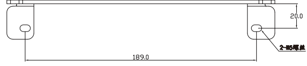
安装板开孔
